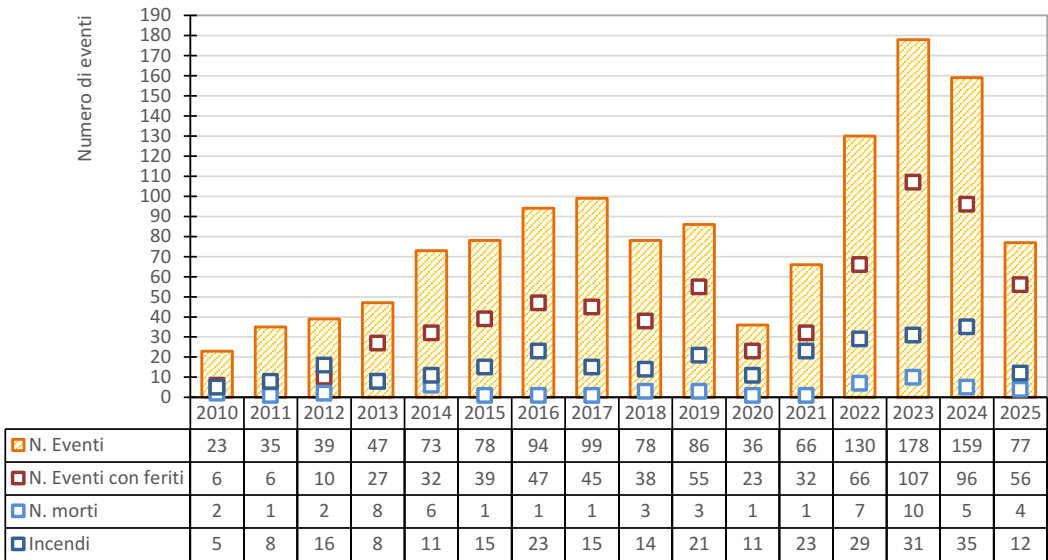
Figura 66: Eventi totali in galleria, di incidenti e/o incendi, correlati alle relative conseguenze
