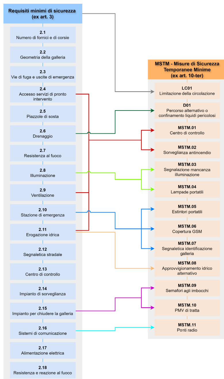
Figura 33: "MSTM-Misure di Sicurezza Temporanee Minime" vs. "Requisiti minimi di sicurezza".
