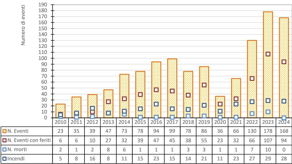
Figura 5 – Eventi totali in galleria, di incidenti e/o incendi, correlati alle relative conseguenze
