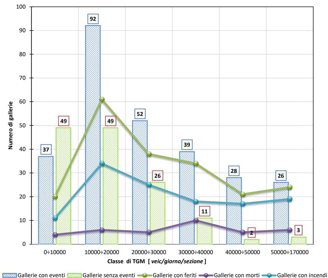
Figura 8 - Classificazione delle gallerie interessate (o meno) dall'incidentalità al variare del TGM per sezione
