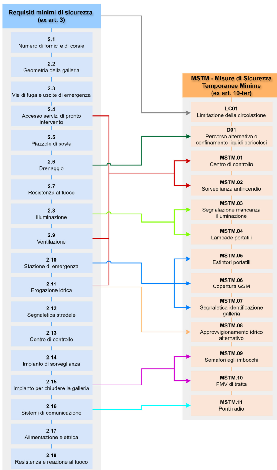
Figura 2 - "MSTM-Misure di Sicurezza Temporanee Minime" vs "Requisiti minimi di sicurezza".
