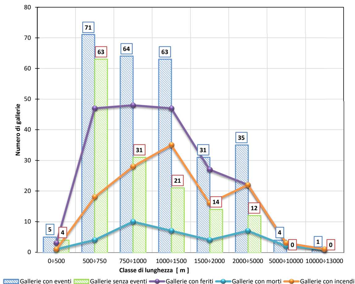
Figura 7 - Classificazione delle gallerie interessate (o meno) dall'incidentalità al variare della lunghezza
