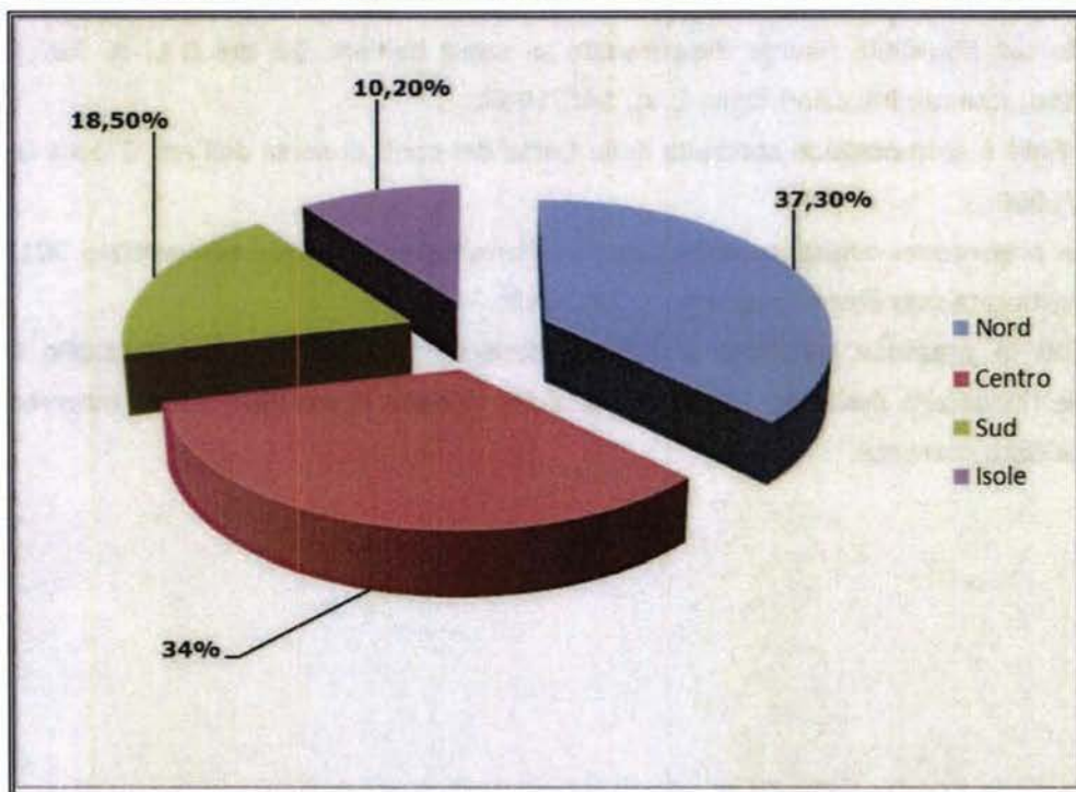
Grafico n. 1 : Percentuale degli iscritti residenti in attività di servizio suddivisi per zone
