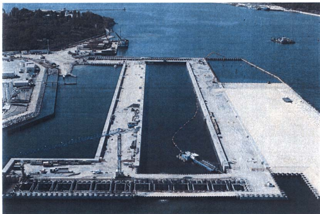
Bocca di Malamocco: In primo piano la porta lato mare della conca di navigazione per grandi navi (centro della foto) che consentirà il transito a imbarcazioni con lunghezza fino a 280 m, larghezza fino a 39 m e pescaggio fino a 12 m. Sulla destra, il terrapieno e la vasca ove verranno ubicati gli impianti e gli edifici tecnologici.
