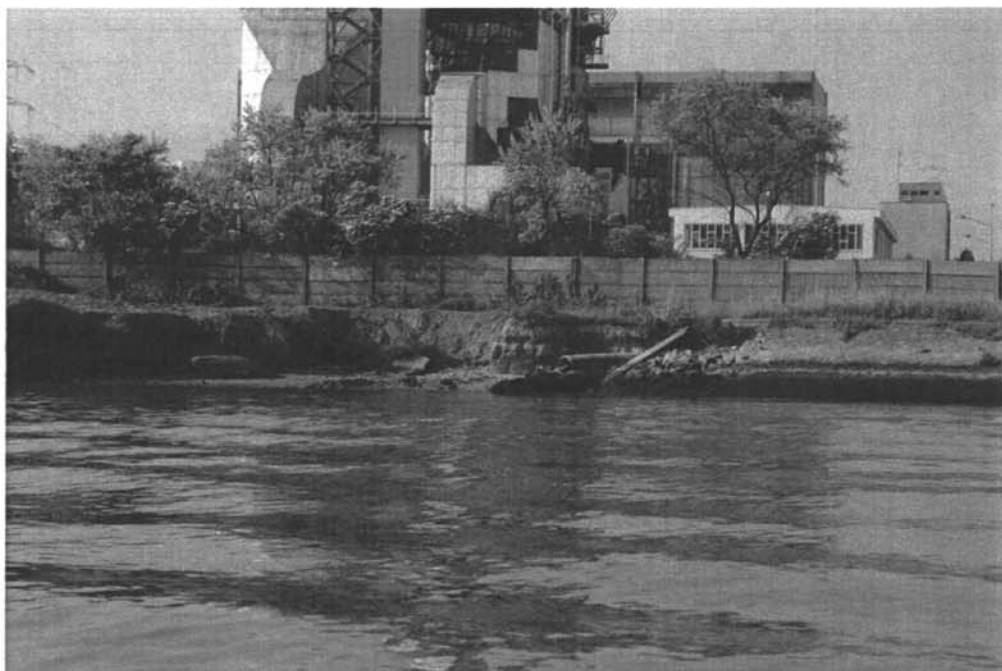
Canale industriale sud sponda sud, area Fassa ex Edison. Stato di fatto di un tratto di marginamento
