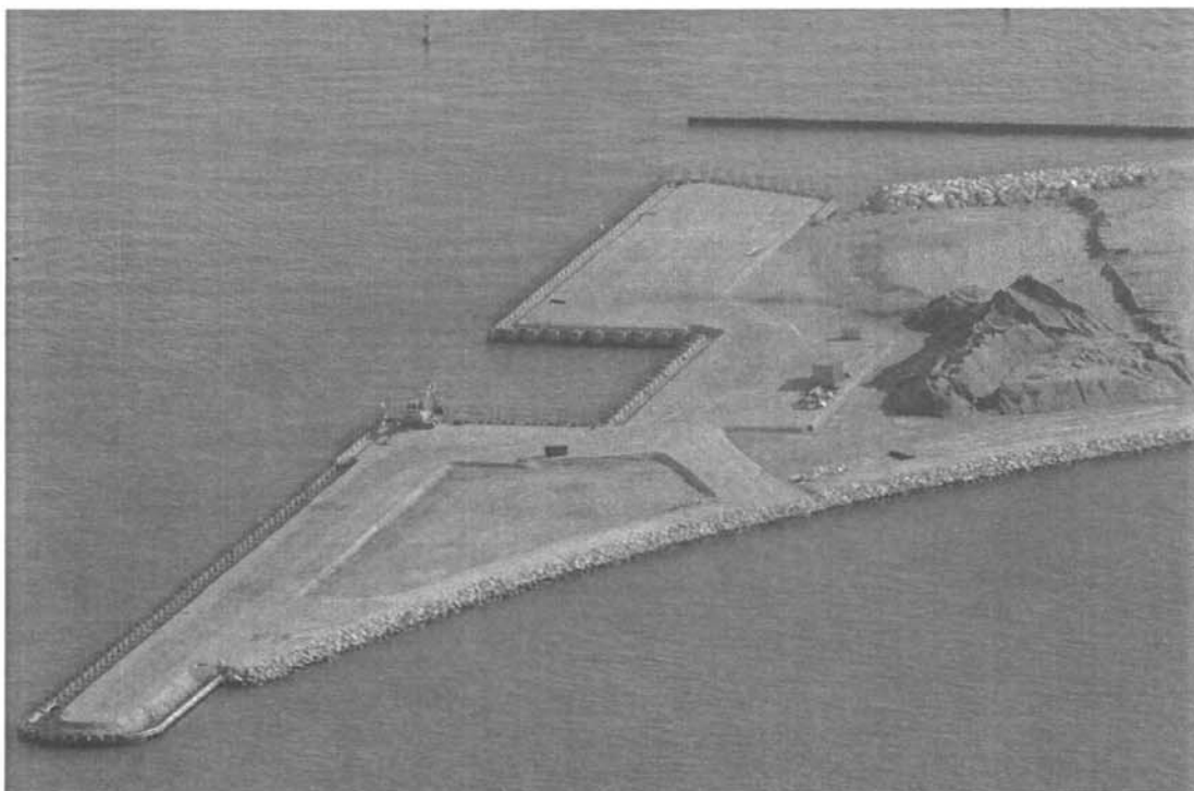
Bocca di Lido : l'isola nuova con al centro della foto il recesso che ospiterà la spalla ovest della barriera di Treporti.
