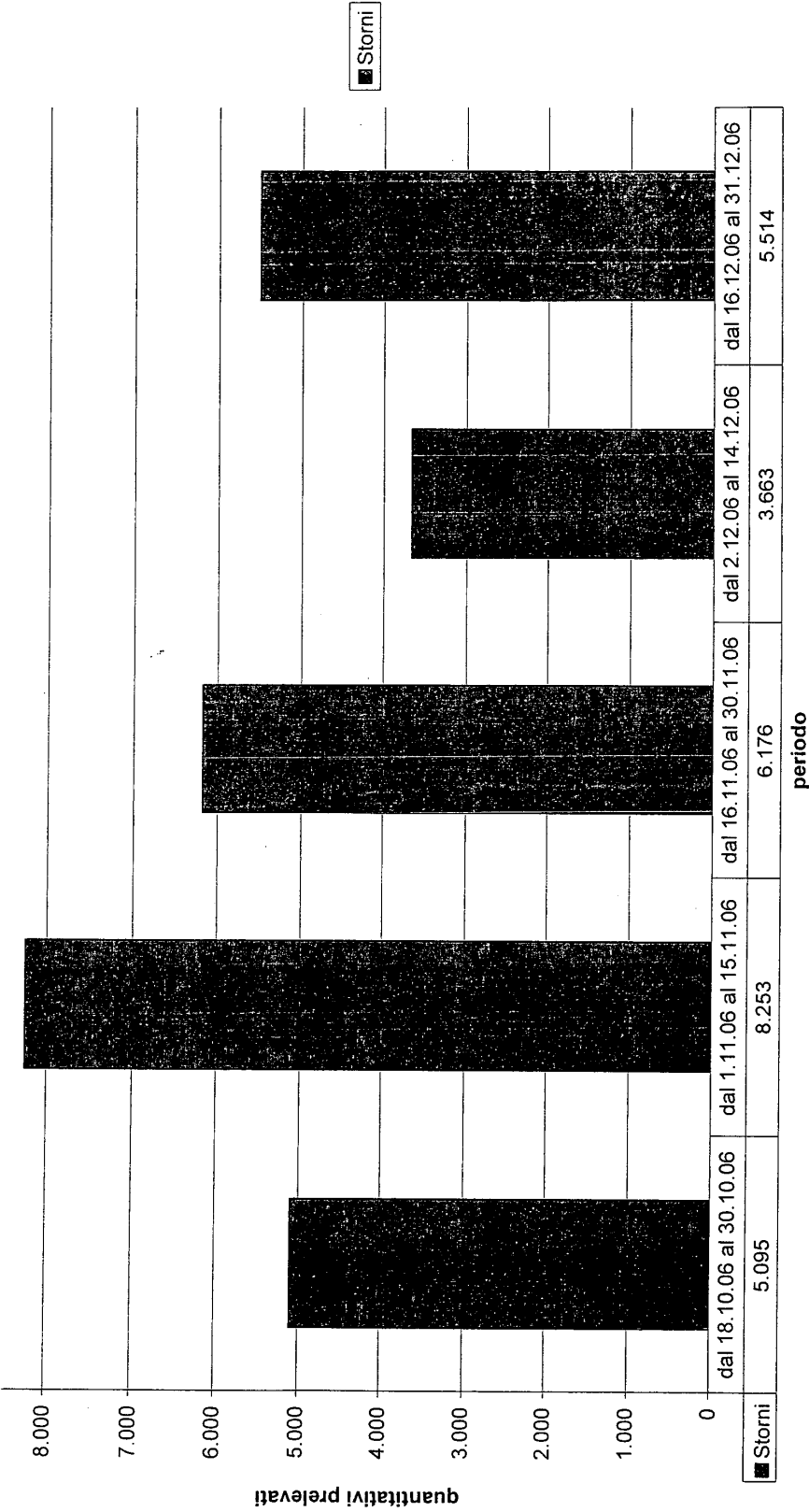
Quantitativi totali di prelievo della specie Storno per quindicina
