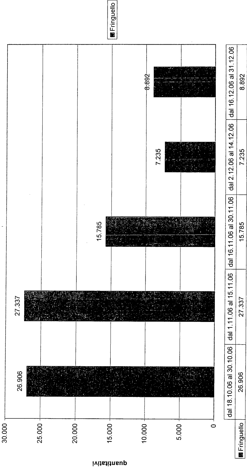
Quantitativi totali di prelievo del Fringuello per quindicina
