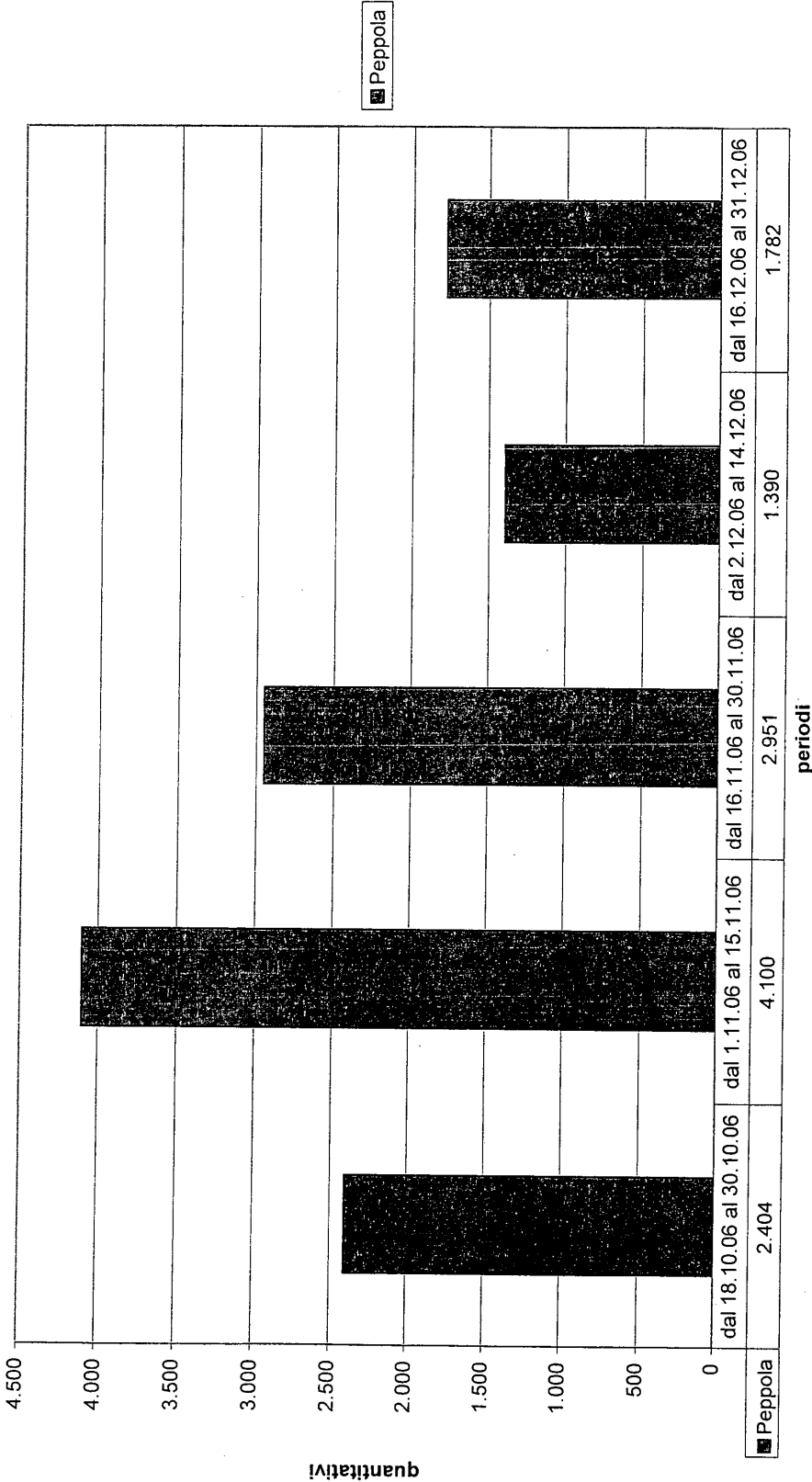
Quantitativi totali di prelievo della specie Peppola per quindicina
