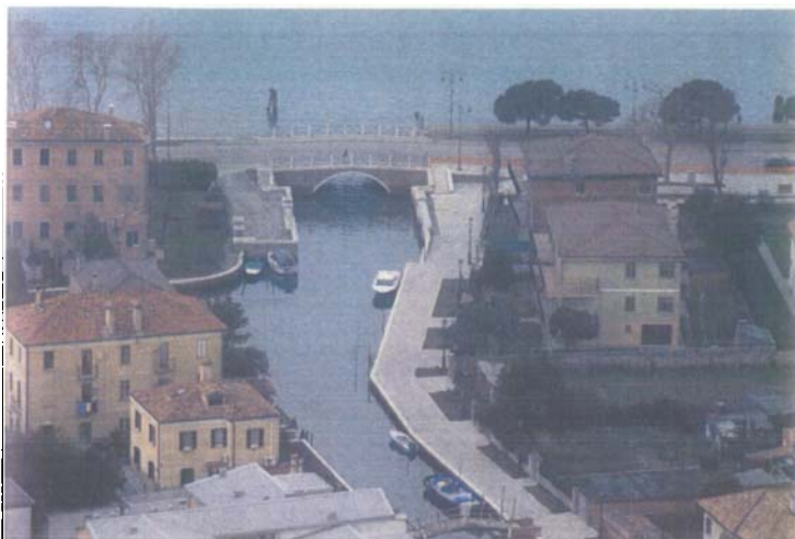
Vista aerea del rio Squero dopo i lavori di sistemazione delle rive
