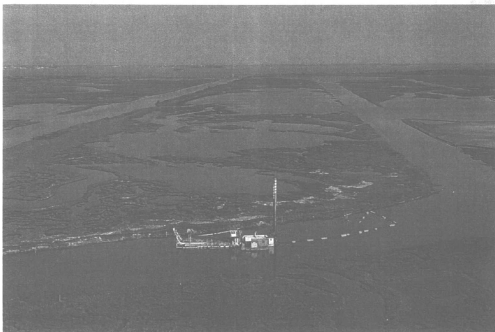
Lago Teneri. Vista aerea della zona di intervento durante i lavori di ripristino della barena.
