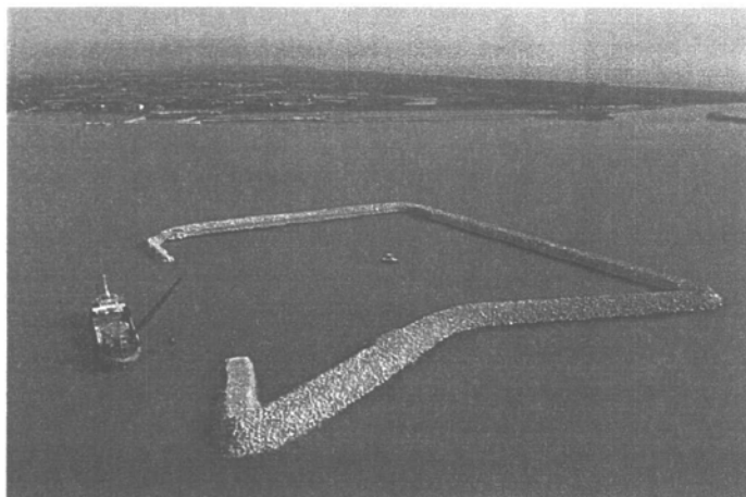
Bocca di Lido – Isola tra S. Nicolò e Treporti 1 a fase
