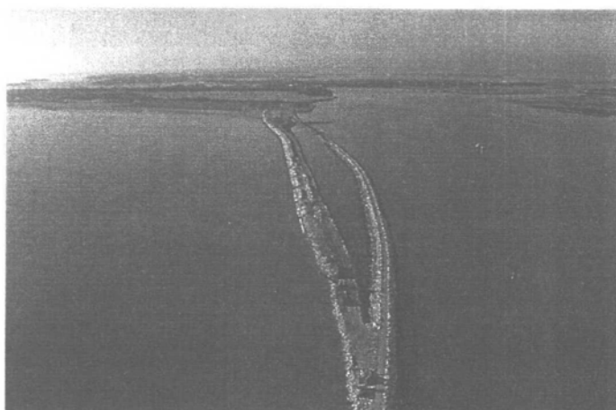
Bocca di Lido- Rinforzo radice del molo sud. Vista aerea della nuova scogliera lato mare.
