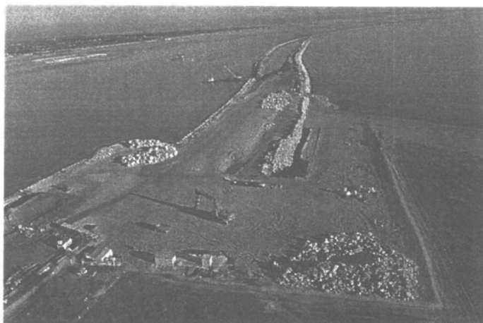
Bocca di Lido - Rinforzo radice del molo sud
