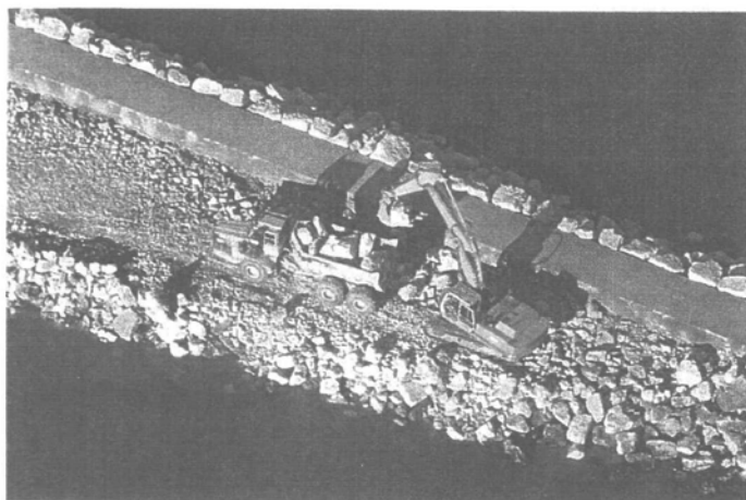
Bocca di Lido- Rinforzo radice del molo sud. Mezzi in opera.
