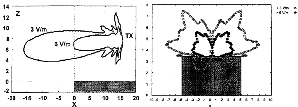
Fig. 31 - Curve di livello di una stazione base macrocellulare (a) e microcellulare (b)
