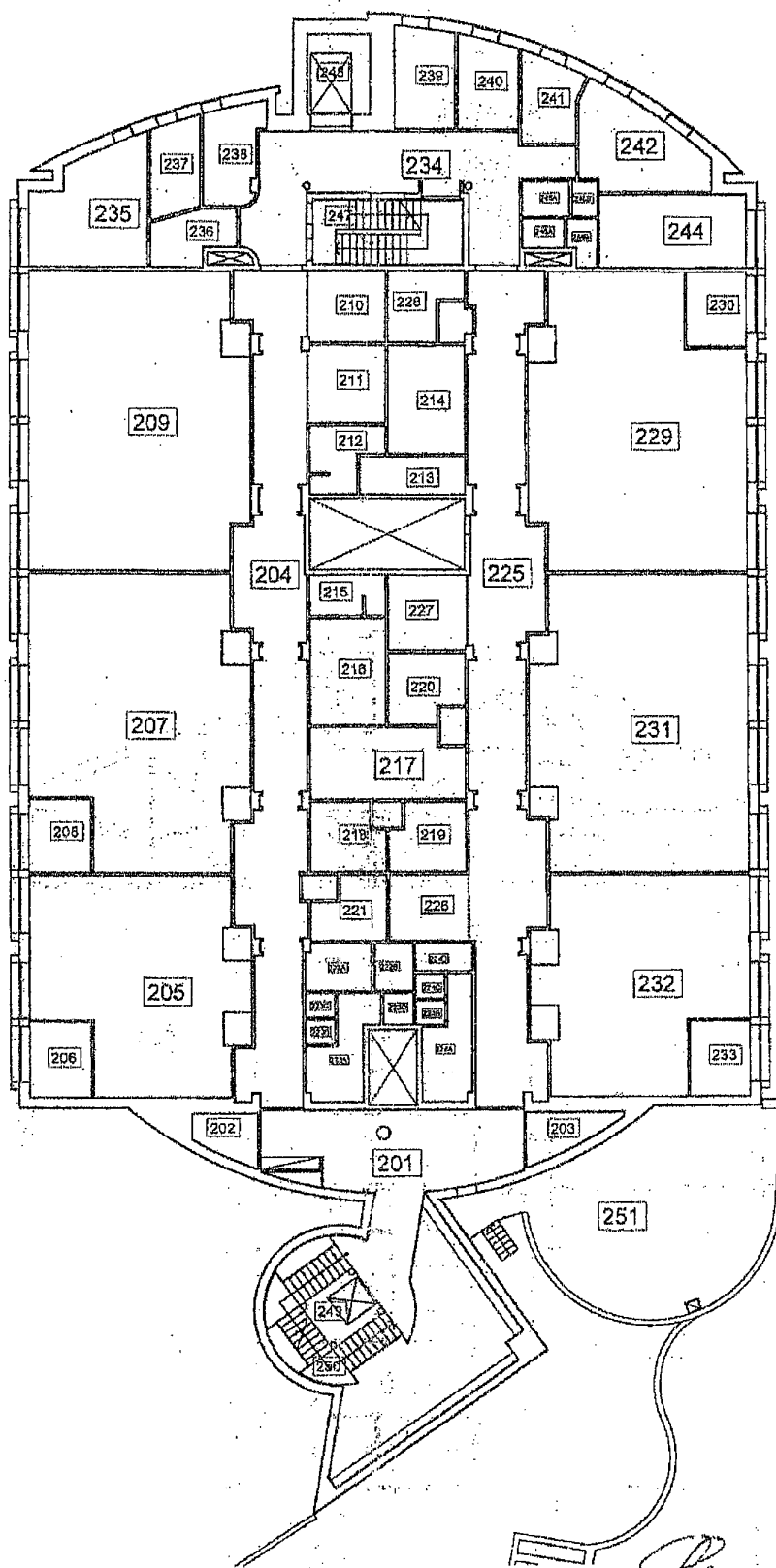
PADRICIANO Edificio W Piano secondo 1:250
