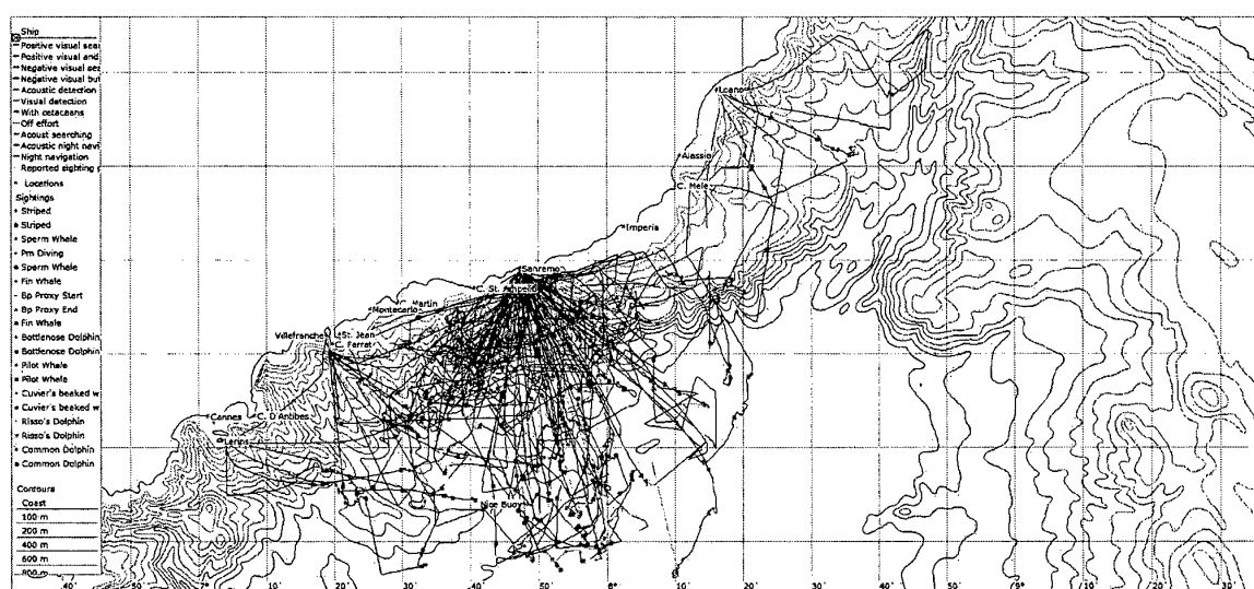
Figura 2. Sforzo di ricerca condotto dall'Istituto Tethys tra il 28 maggio e il 28 settembre 2019, e gli avvistamenti effettuati di 6 diverse specie di cetacei.
