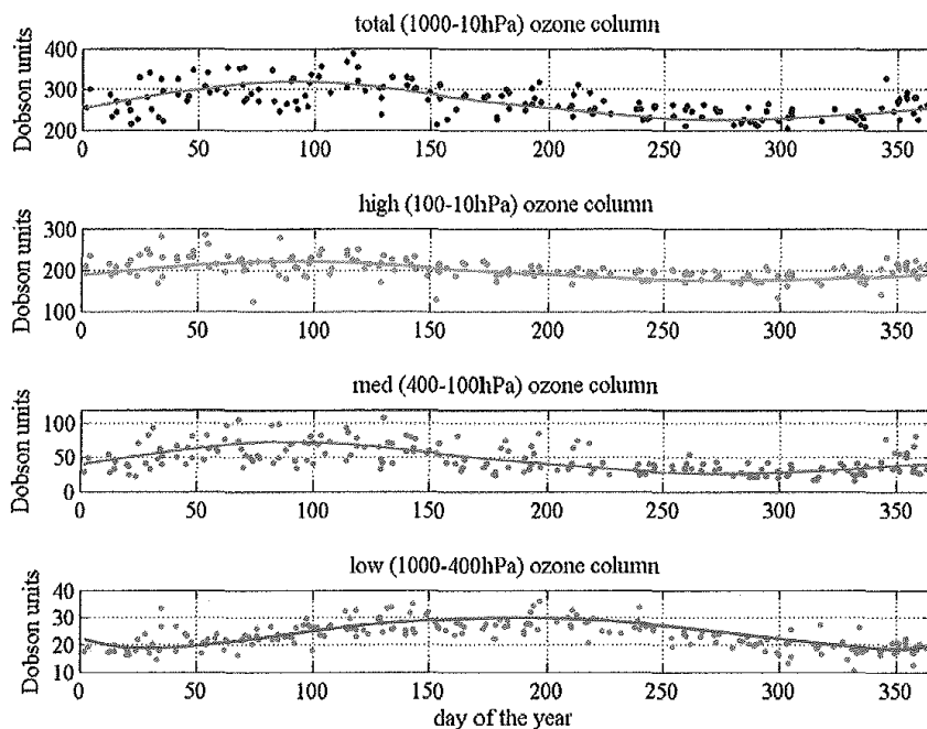
Figura 1. Le misure del contenuto colonnare di ozono sul sito dell'Osservatorio Atmosferico di CETEMPS. "total" si riferisce alla contenuto totale della colonna di ozono, senza correzioni, "high" è il contenuto di ozono nella stratosfera, "med" è il contenuto di ozono nella troposfera libera, infine "low" è rappresentativo del contenuto di ozono nello strato limite planetario.
