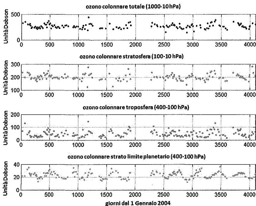
Figura 4. Il contenuto colonnare di ozono in diversi strati dell'atmosfera; dal pannello in basso a quello verso l'alto: nello strato limite planetario, nella troposfera libera, nella stratosfera e la colonna totale. Le serie temporali partono dal 1 Gennaio 2004 e includono tutte le osservazioni del 2015.
