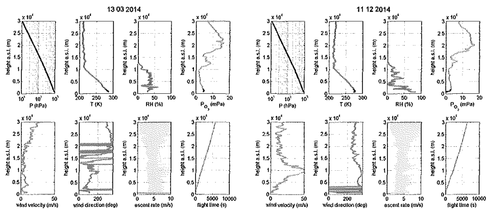
Figura 2. Due diversi ozono-sondaggi sul sito dell'Osservatorio Atmosferico di CETEMPS. Il sondaggio primaverile (13 Marzo 2014) mostra un contenuto di ozono stratosferico maggiore rispetto all'ozono-sondaggio invernale (11 Dicembre 2014).
