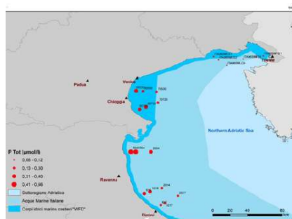
Figura 2.14: Concentrazioni di Fosforo nelle coastal waters dell'Alto Adriatico (2012-2015)
