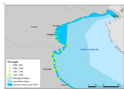
Figura 2.17: Concentrazioni di clorofilla "a" nelle coastal waters dell'Alto Adriatico (2012-2015)
