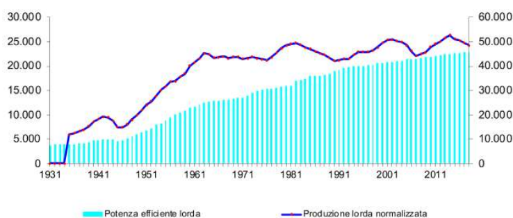
Figura 4.12: Produzione idroelettrica lorda e capacità installata in Italia fino al 2018
