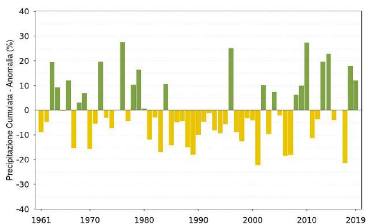
Figura 4.4: Serie delle anomalie medie in Italia, espresse in valori percentuali, della precipitazione cumulata annuale rispetto al valore normale 1961-1990
